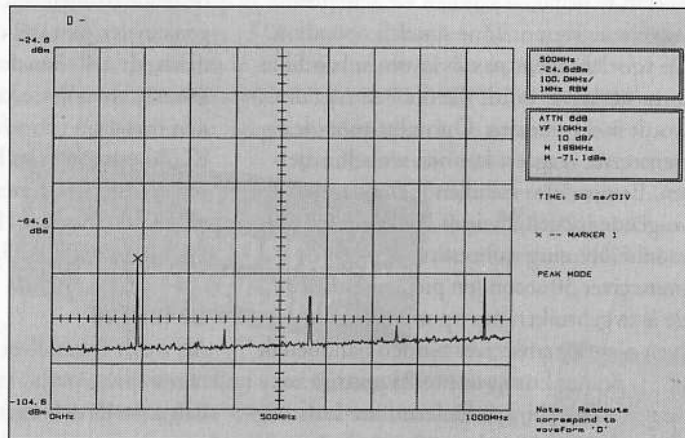
Figuur 4: Het spectrum VHF-band (RX).
